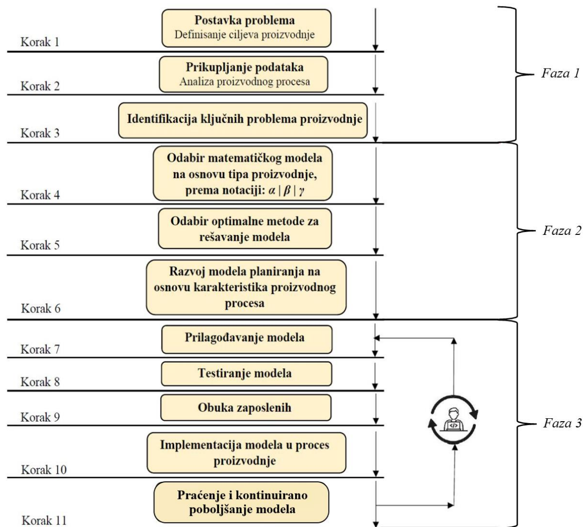
Slika 5.3 Garfički prikaz osnovnih koraka pri razvoju modela
