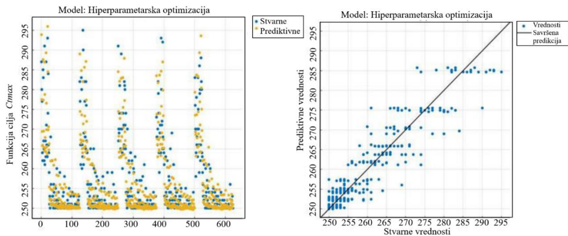
Slika 6.7 Grafički prikaz dobijenih rezultata korišćenjem modela Bajesove optimizacije
