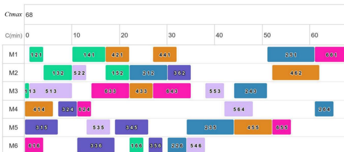
Slika 5.32 Grafčki prikaz delimične fleksibilnosti i rasporeda proizvodnog procesa
