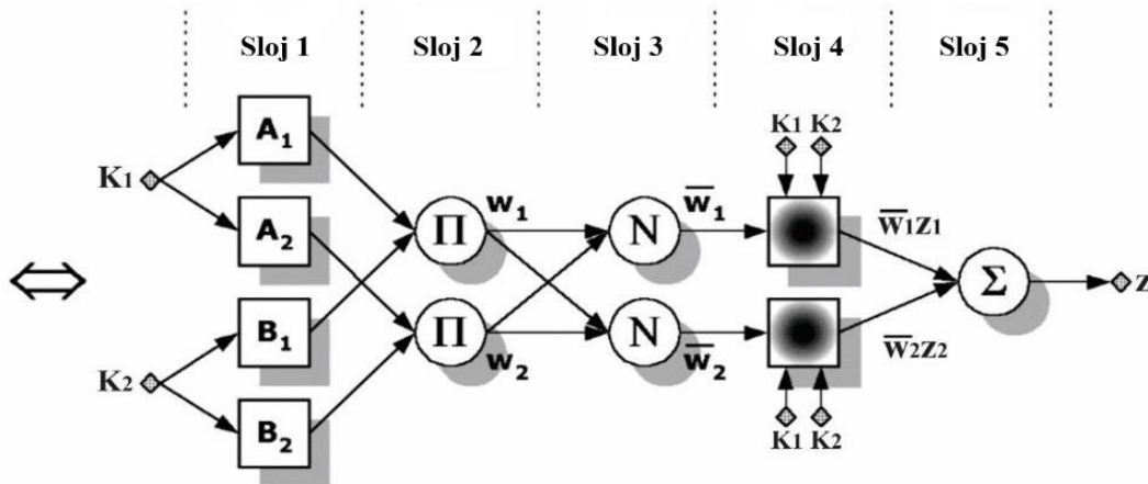
Slika 4.22 Osnovna struktura ANFIS sistema
