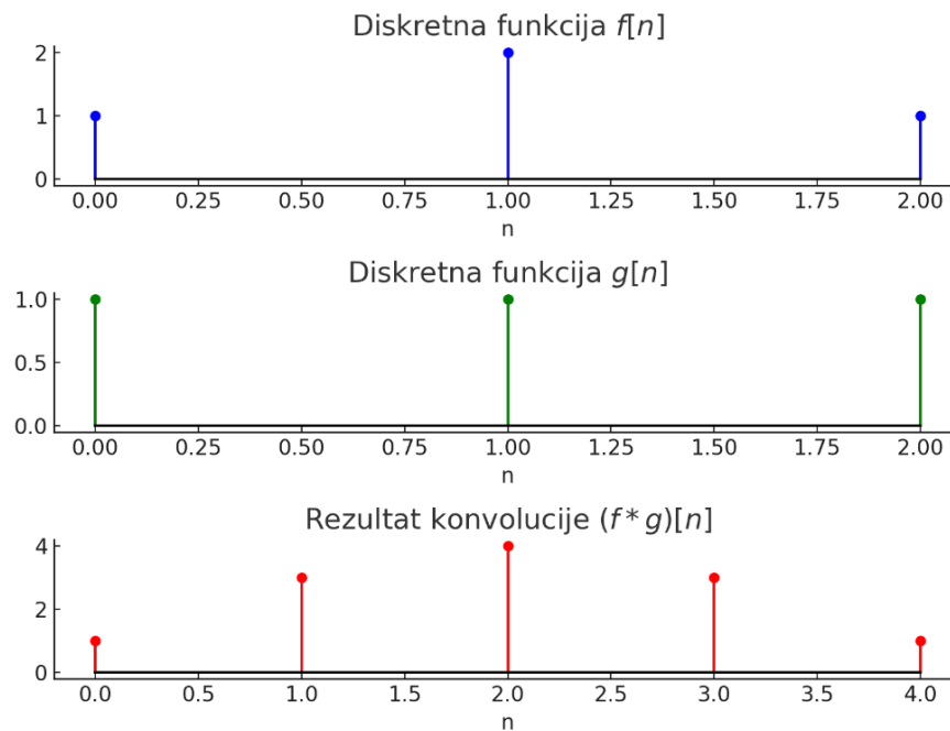
Slika 4.11 Grafički prikaz dobijenih rezultata primenom diskretne konvolucije
