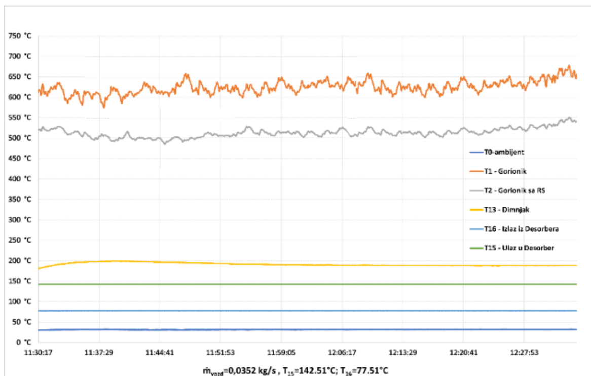
Слика 3.80. Расподела температура у ГВВ и кроз десорбер АП, 30 kW горионик, I – брзина вентилатора
