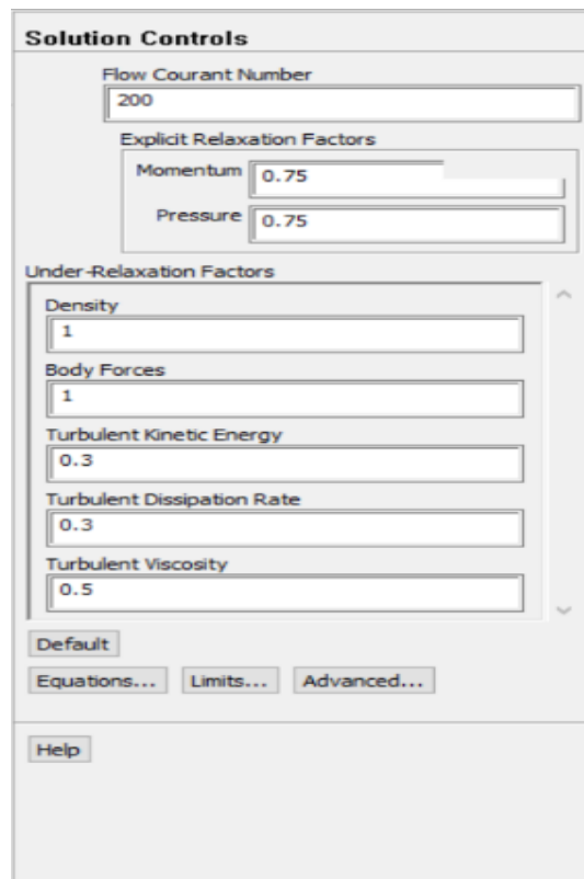
Слика 4.11. Приказ иницијалних подешавања у софтверу
