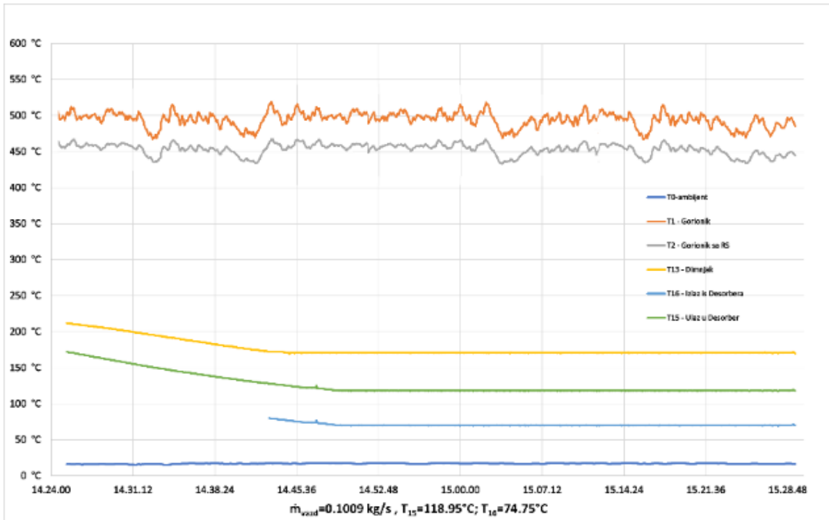
Слика 3.73. Расподела температура у ГВВ и кроз десорбер АП, 30 kW горионик, III – брзина вентилатора
