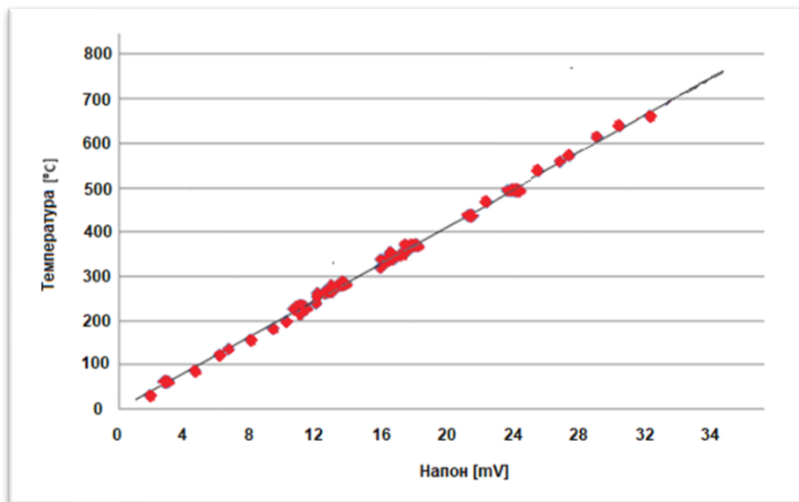
Слика 3.52. Баждарење термопарова
