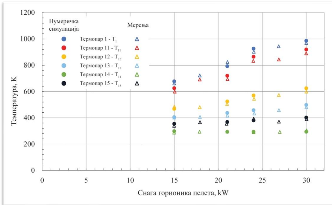
Слика 4.28. Поређење резултата мерења и нумеричких симулација температуре продукта сагоревања на изабраним локацијама T_1 , T_{11} , T_{12} и T_{13} , као и температуре ваздуха T_{14} и T_{15} , у зависности од снаге горионика, у зимском режиму ( t_v \sim 7^\circ\text{C} ), при протоку ваздуха од 0.170\text{ kg/s}
