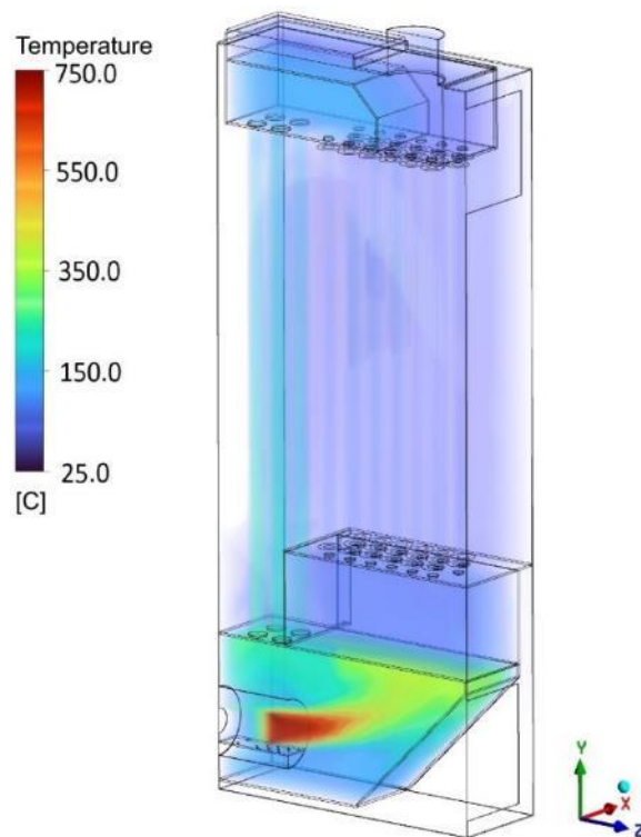
Слика 4.23. Температурско поље по запремини ГВВ
