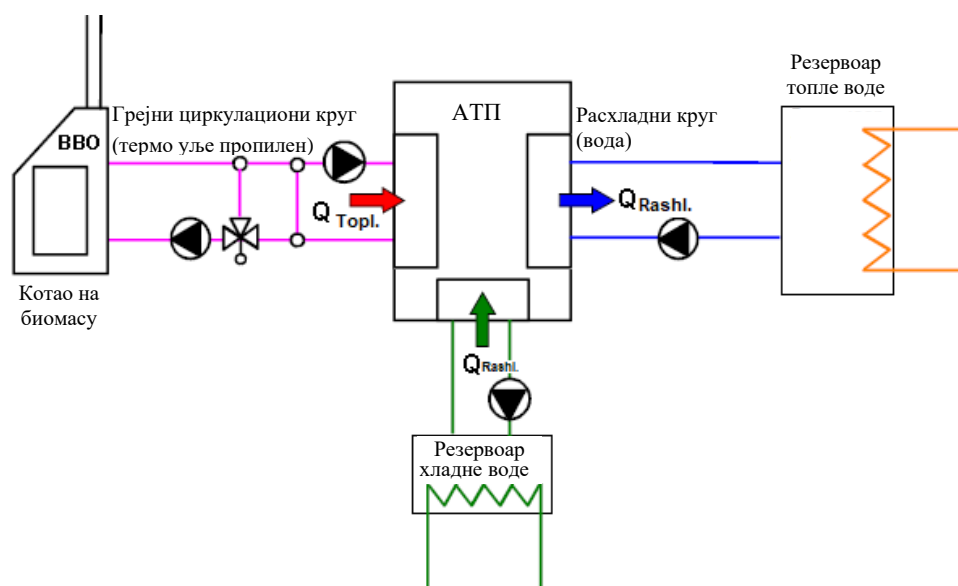
Слика 2.5. Принципијелна шема апсорционог једностапеног циклуса на биомасу као генератор топлоте у десорберу АТП - BioAWP
