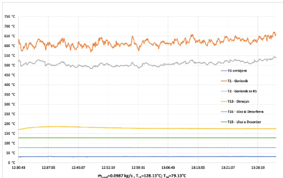
Слика 3.82. Расподела температура у ГВВ и кроз десорбер АПГ, 30 kW горионик, III – брзина вентилатора
