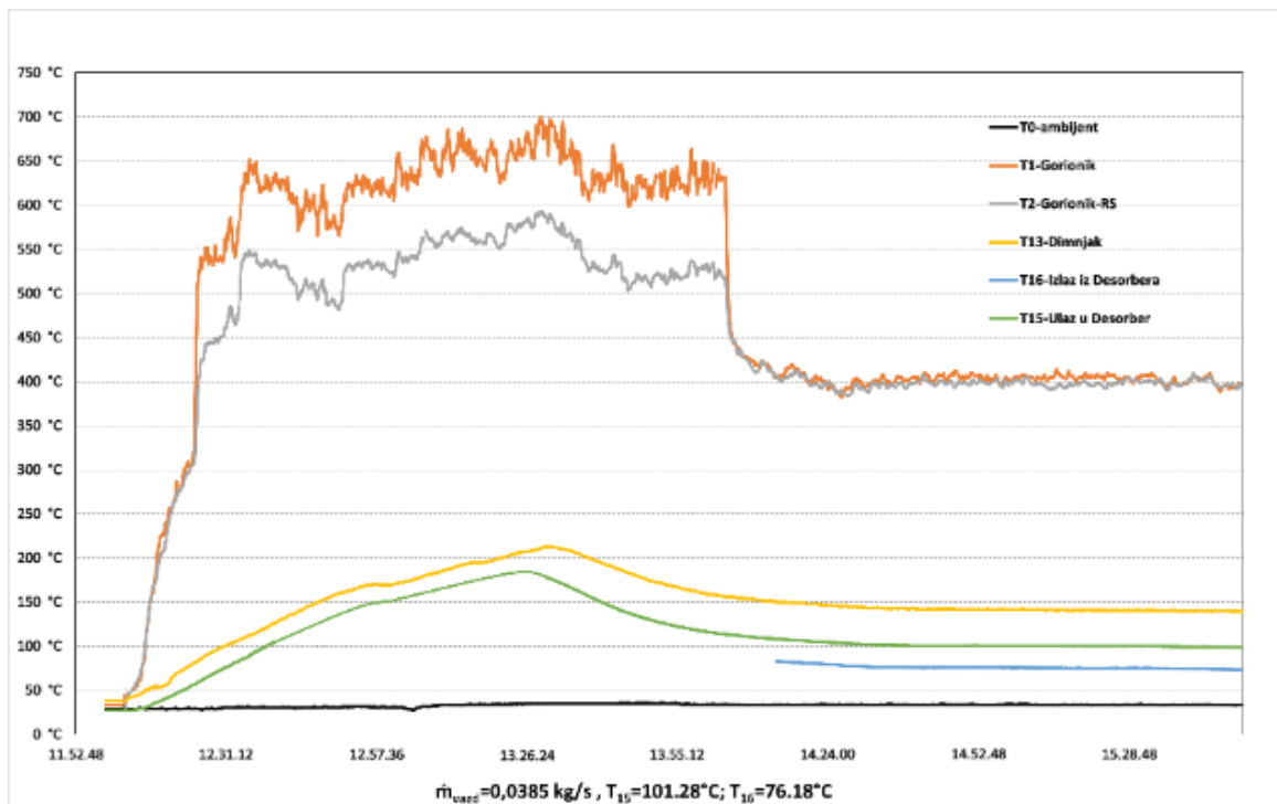
Слика 3.74. Расподела температура у ГВВ и кроз десорбер АП, 15 kW горионик, I – брзина вентилатора
