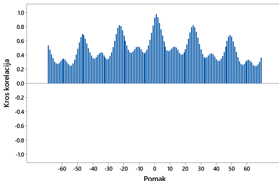
Слика 5.22 Приказ крос-корелационе функције за топлотно оптерећење и температуру повратног вода примара, подаци из новосадског СДГ
