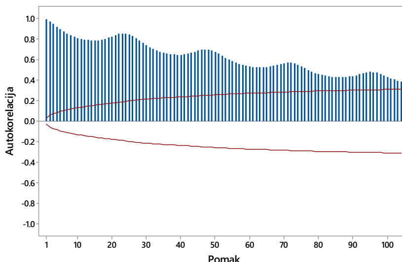
Слика 5.24 Приказ аутокорелационе функције за спољну температуру, подаци из новосадског СДГ
