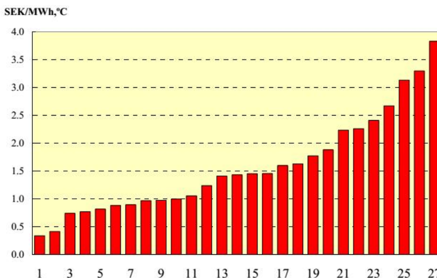
Слика 2.36 Уштеда у SEK/MWh произведене топлотне енергије у СДГ за снижење температуре поврата од 1 0 C за 27 СДГ у Шведској за период од 1996-2010 [Petersson/Werner]
