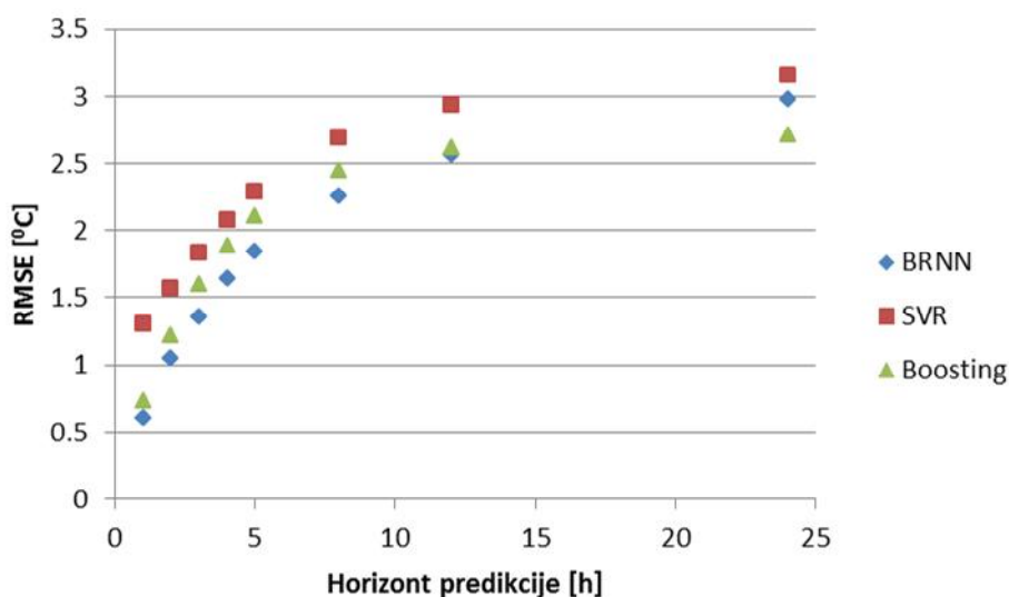
Слика 5.28 Упоредни приказ резултата предикције, новосадски СДГ, улазне променљиве - спољна температура са временским кашњењем од 1 – 48h
